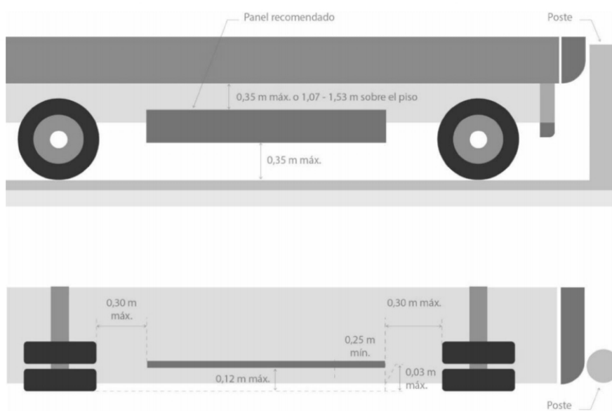
Figura 1. Características recomendadas del salvaguarda
